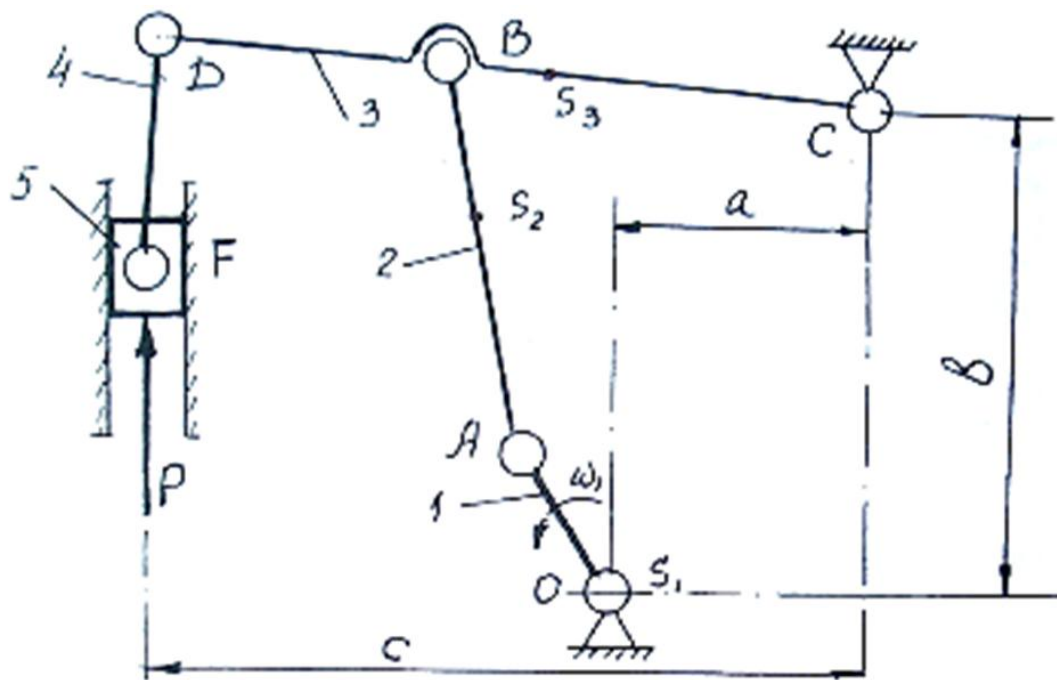
Кинематическая схема механизма
